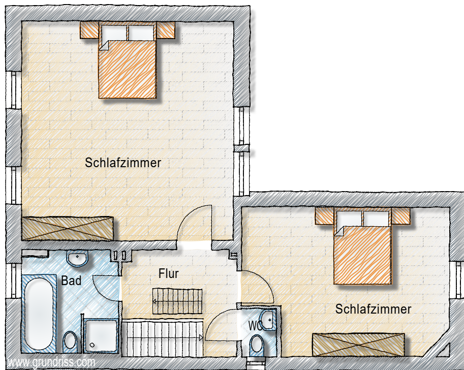
Obergeschoss
