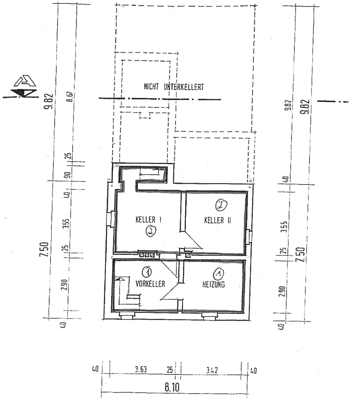
KELLERGESSCHOSS
